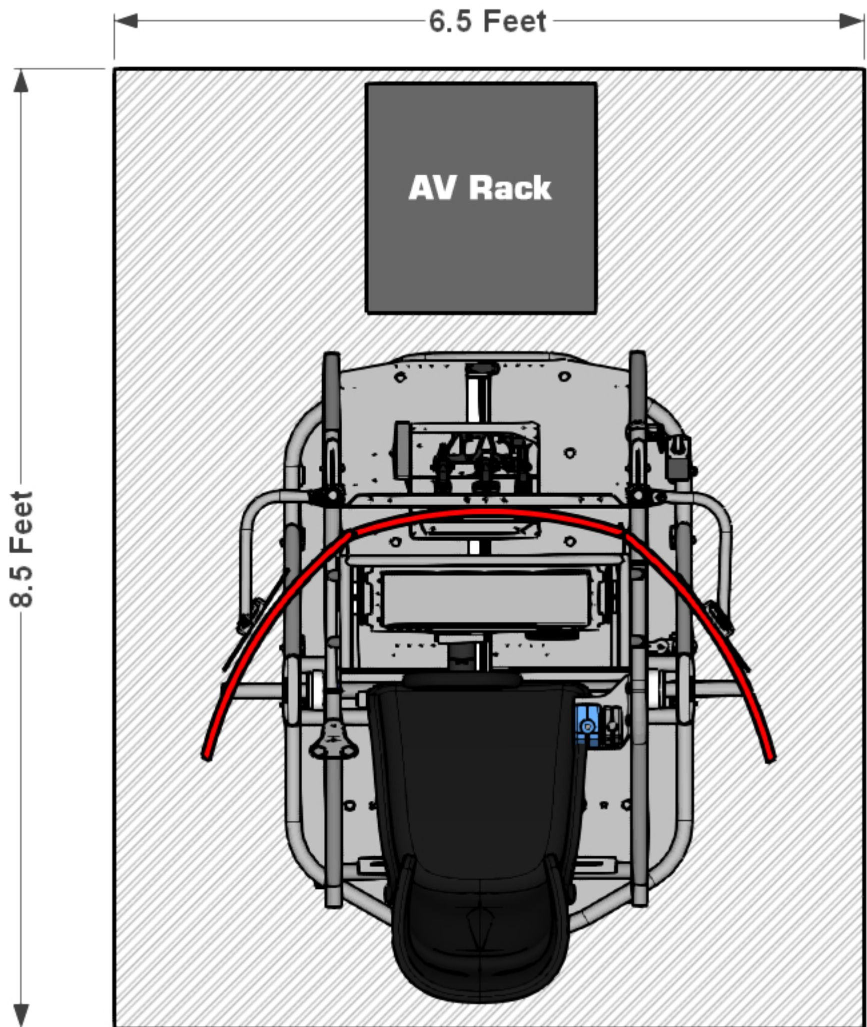
APEX CT | Triple Curved 32" | Front AV Rack Dimensions
