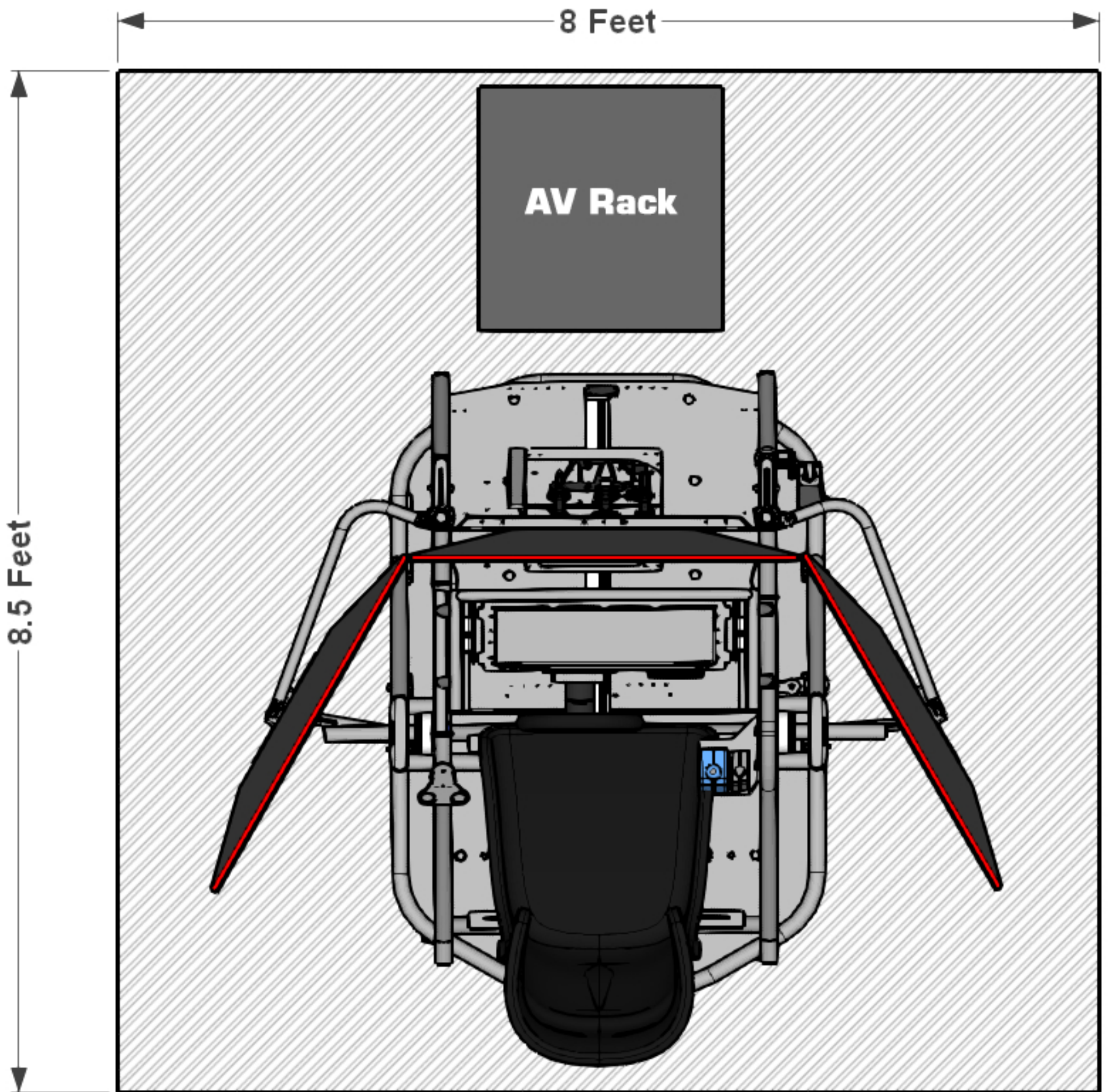
APEX CT | Triple Curved 32" | Front AV Rack Dimensions
