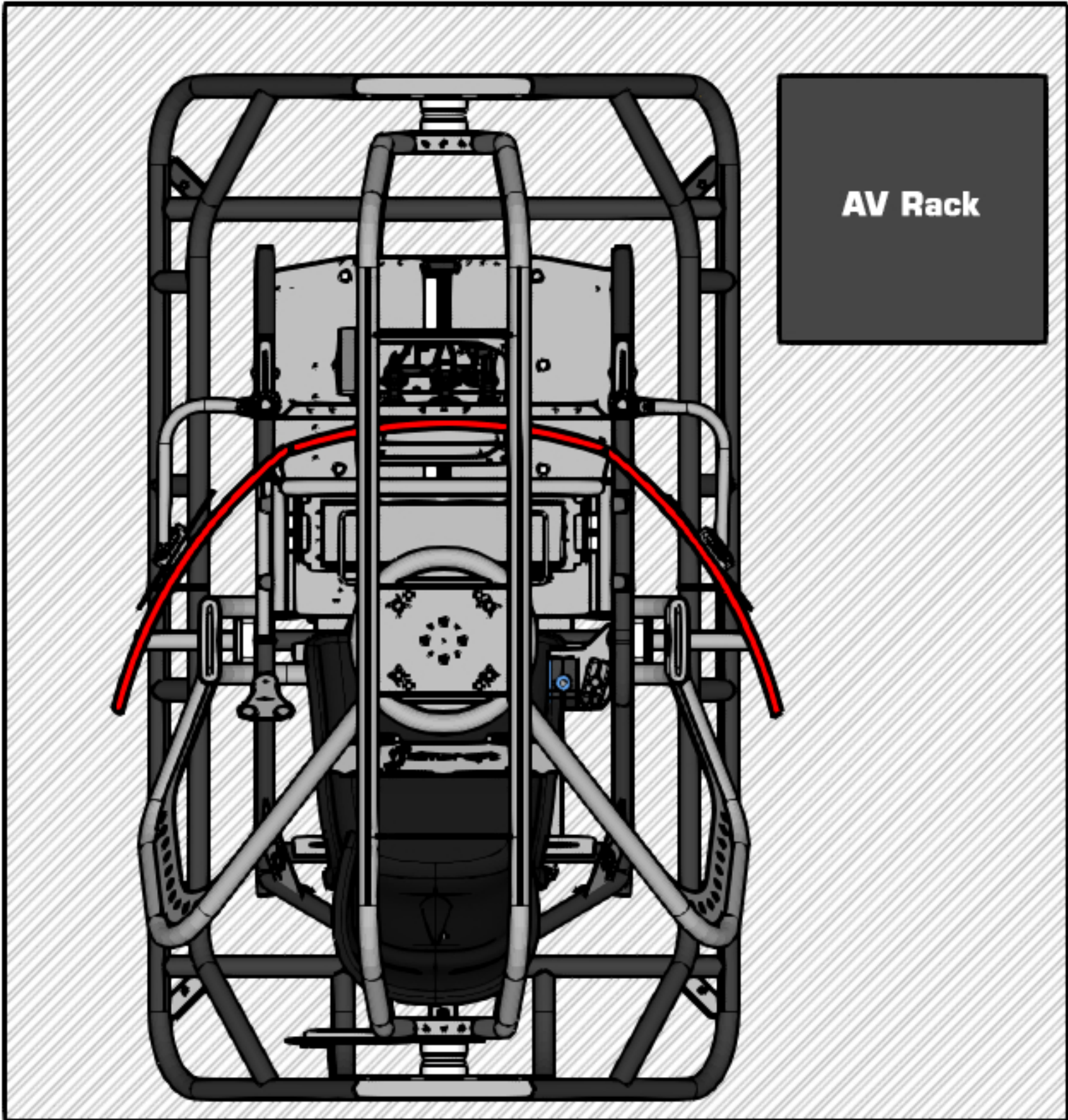
APEX GT | Triple Curved 32" | Side AV Rack Dimensions
