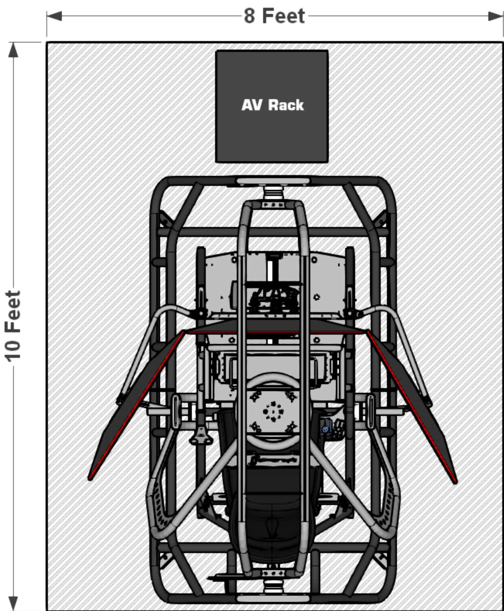
APEX GT | Triple Flat 43" | Front AV Rack Dimensions
