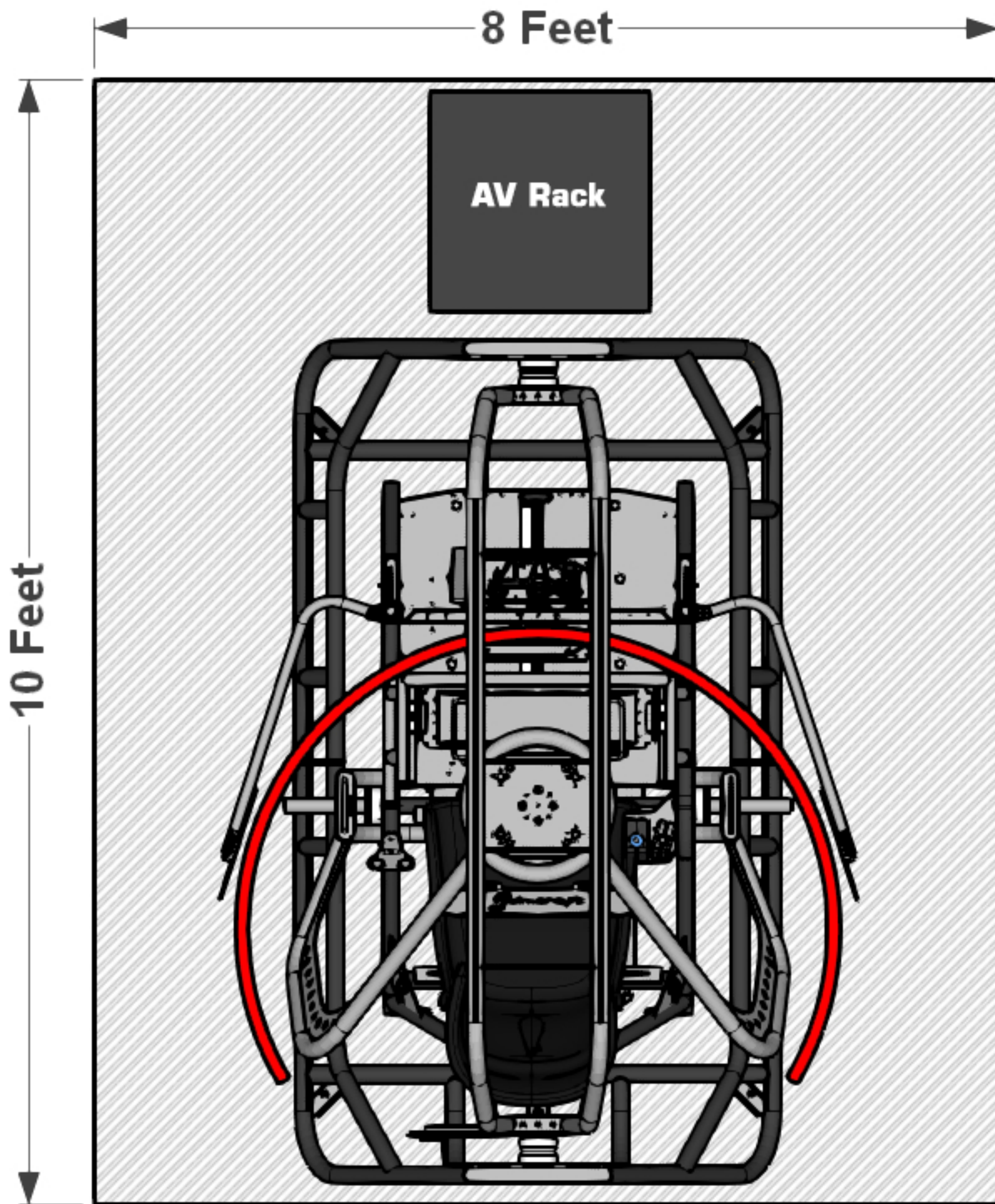
APEX GT | Triple Curved 45" | Front AV Rack Dimensions
