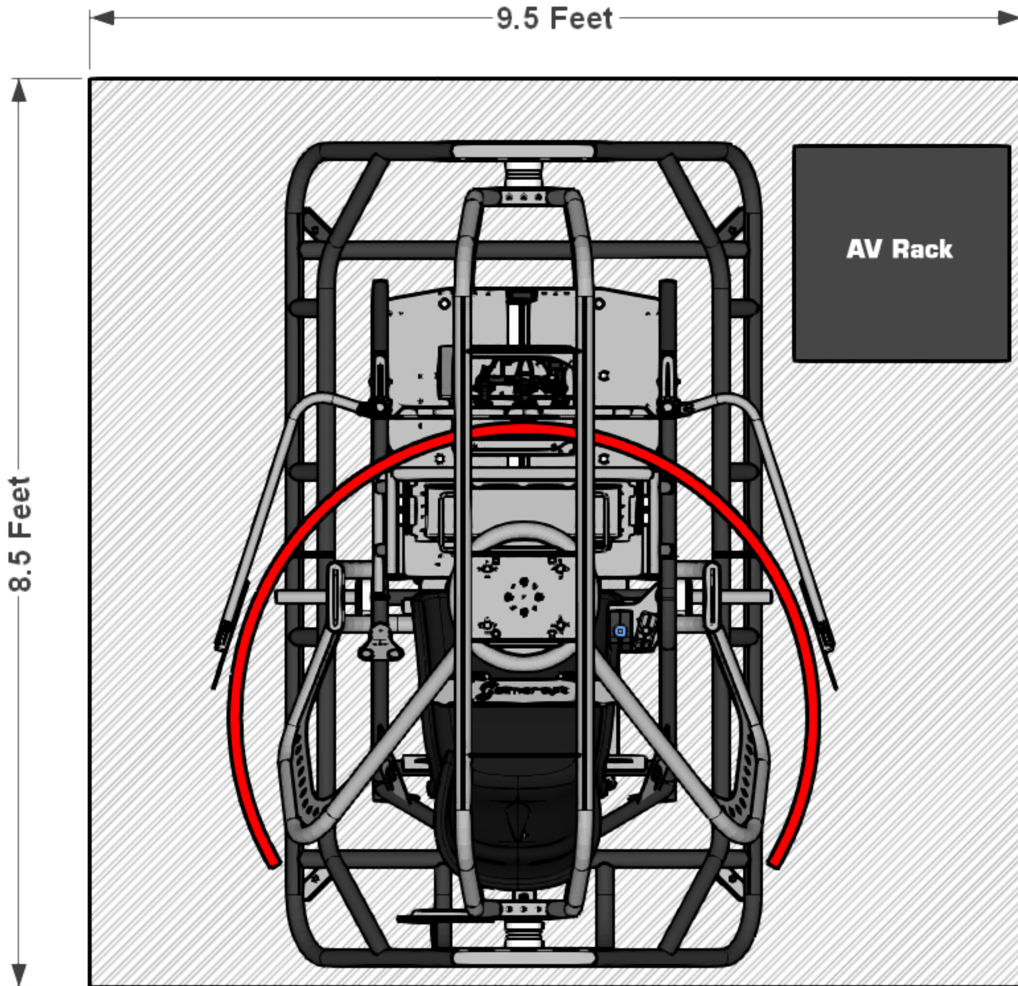
APEX GT | Triple Curved 45° | Side AV Rack Dimensions
